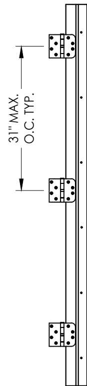
HINGE JAMB
